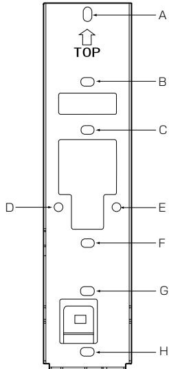
【壁掛け金具穴位置寸法】
